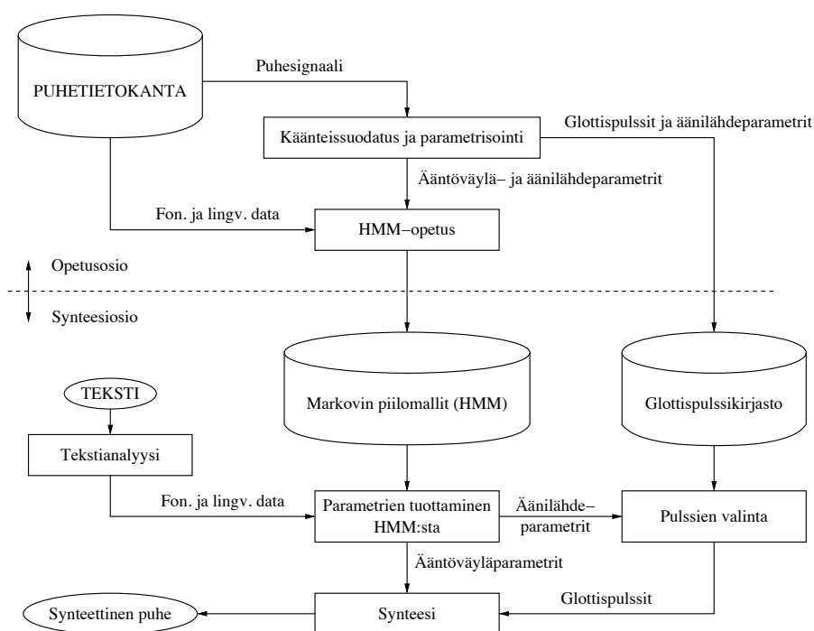
Kuva 1: Puhesynteesijärjestelmän rakenne.
