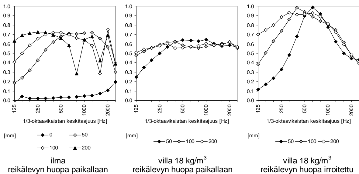
Kuva 8. Taustamateriaalin paksuuden [mm] vaikutus kipsireikälevyn Knauf Belgravia Q1 absorptiosuhteeseen. Taustamateriaalin ja reikälevytuotteessa valmiina olevan huovan status on mainittu kuvan alla. Reikälevyn rei'itysprosentti on 16 % ja reikäkoko 12 \times 12 \text{ mm} .
