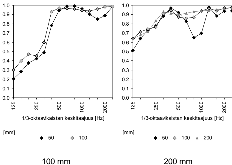
Kuva 2. Lasivillan paksuuden [mm] vaikutus absorptiosuhteeseen eri alaslaskulla, kun tiheys on 18 kg/m 3 . Alaslasku on mainittu kuvan alapuolella.
