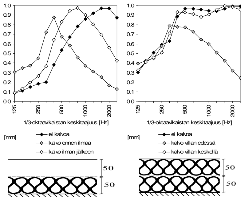
Kuva 7. Kalvon paikan vaikutus absorptiosuhteeseen monikerrosrakenteella kun reikälevyn reijän halkaisija on 4 mm ja rei'itysprosentti on 25 %. Villan tiheys oli 18 \text{ kg/m}^3 .
