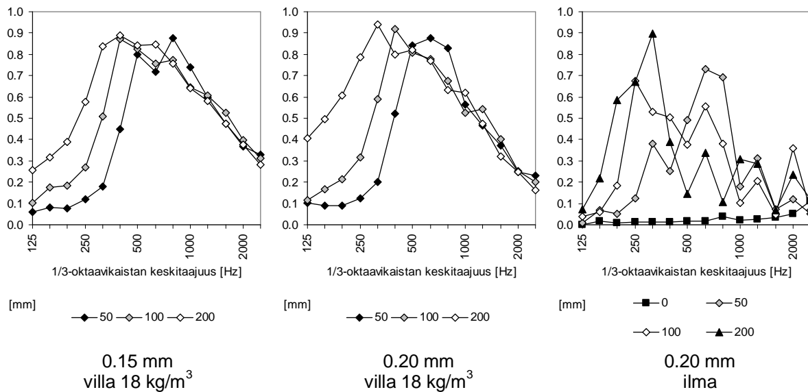
Kuva 6. Höyrynsulkumuovin absorptiosuhde eri paksuisilla taustamateriaaleilla. Alla on mainittu kalvon paksuus ja taustamateriaali. Pelkän lasivillan absorptiosuhde esitettiin kuvassa 2.
