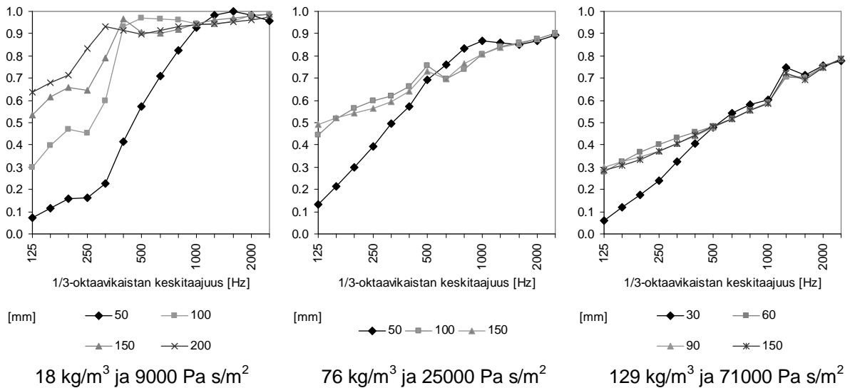
Kuva 1. Lasivillan paksuuden [mm] vaikutus absorptiosuhteeseen. Tiheys ja virtausresistiivisyys on mainittu kuvan alla.
