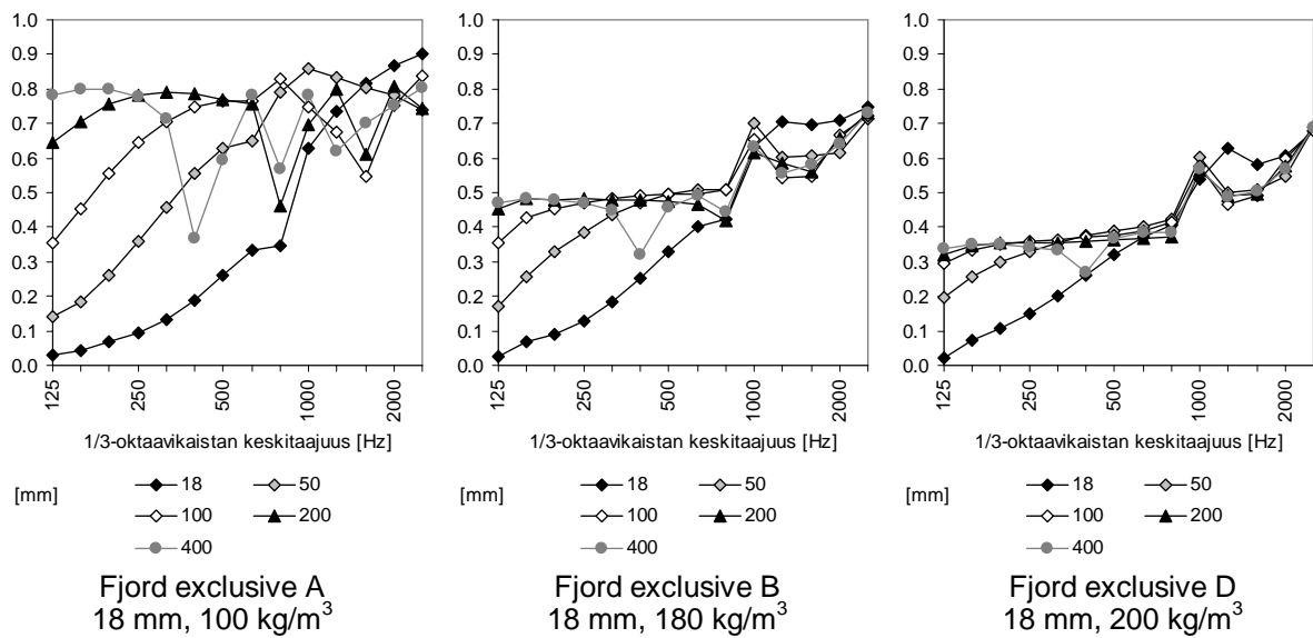
Kuva 3. Alaslaskun vaikutus pinnoitettu kivivillan absorptiosuhteeseen. Kuvan alla on mainittu tuotteen nimi, paksuus ja tiheys.
