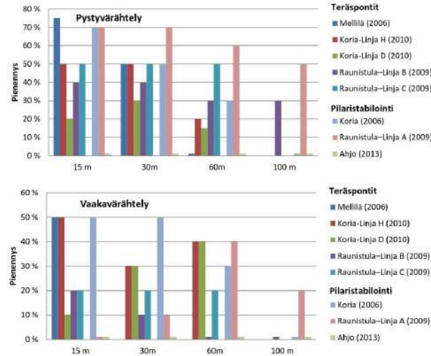
Kuva 5. Yhteenveto värinäesteiden vaikutuksista aikaisemmissa selvityksissä eri etäisyydellä radasta. Ahjon kohde on toteutetun vaimennusrakenteen ja maaperäolosuhteiden osalta jonkin verran muista poikkeava [3].
