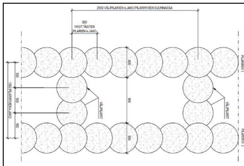
Kuva 2. Pilarit sijoitettiin siten, että stabilointirakenne muodostuu kahdesta pituussuunnaisesta seinästä sekä niiden välisistä poikittaisista seinistä. Seinän pituussuunnassa pilariväli on 500 mm niin että vierekkäiset pilarit leikkaavat toisiaan 100 mm.
